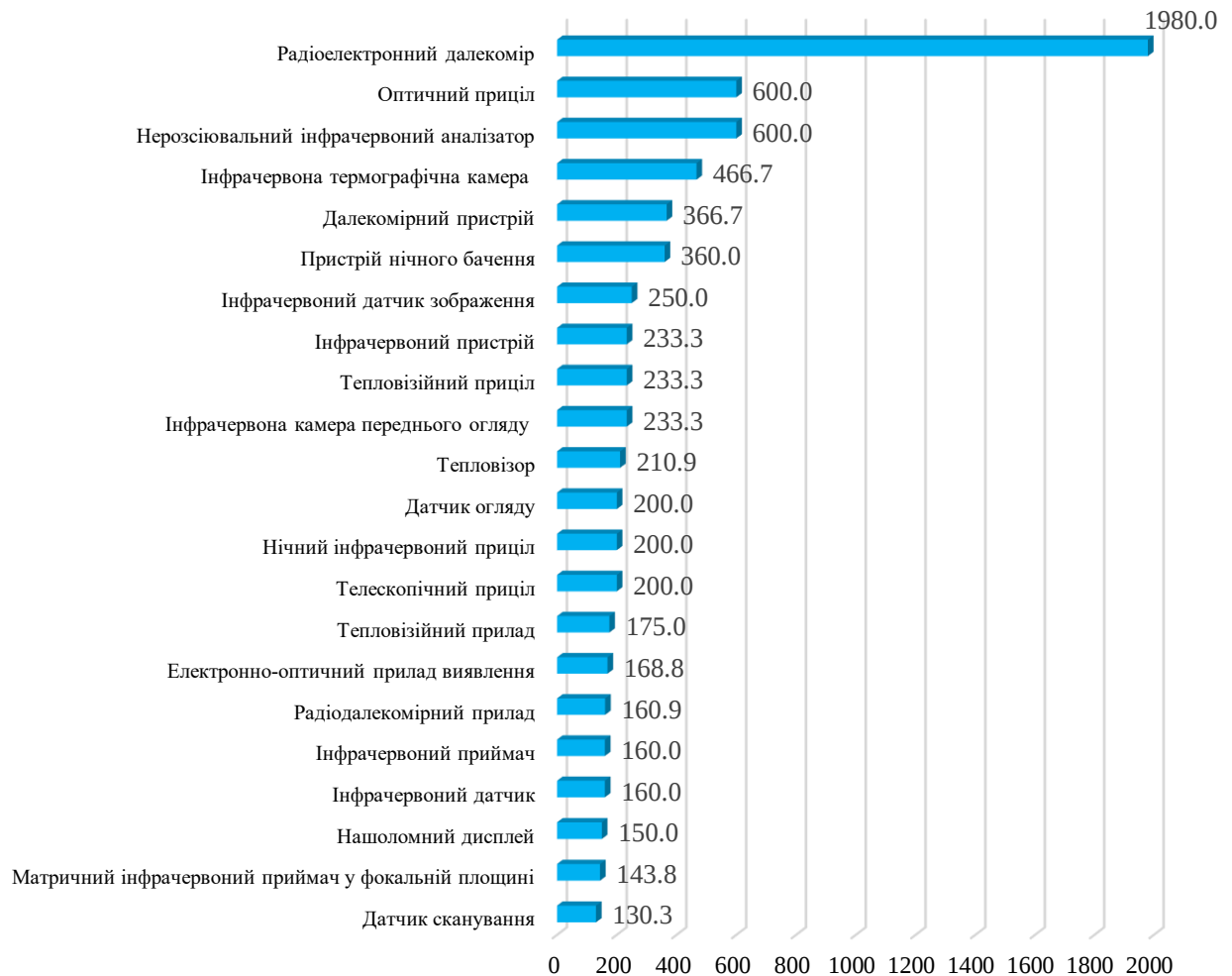
Рис. 2.5 Напрями за темпом публікаційної активності за видом «Оптико-електронні пристрої інфрачервоного діапазону спектру» у 2019-2023 рр., %
